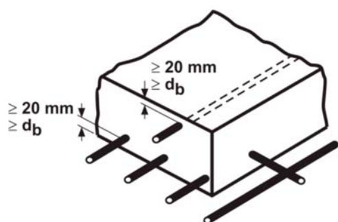
(c) Losas no expuestas al aire libre ni en contacto con el suelo, con d_b \leq 32\text{ mm}
