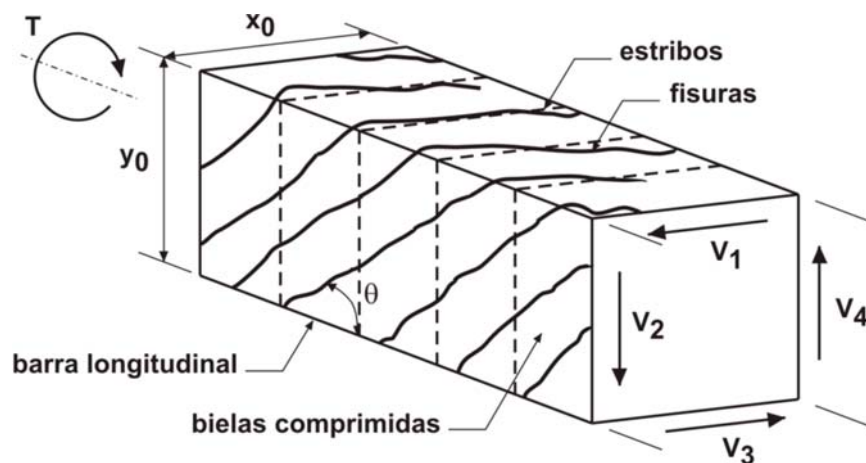
Figura 11.6.3.6.a) Analogía del reticulado espacial para torsión.
