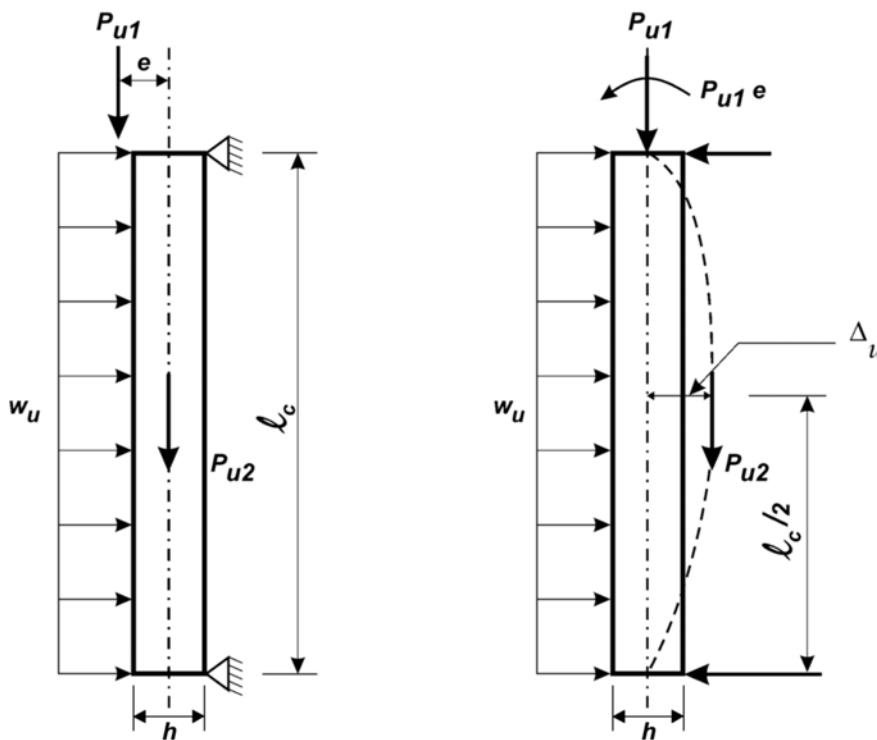
Figura 14.8. Diseño alternativo para tabiques esbeltos
