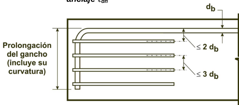
Figura 12.5.3.b.) Disposición de los estribos tanto abiertos como cerrados, ubicados en forma paralela a la barra o alambre que se está anclando, con las separaciones que se indican a lo largo de la longitud de prolongación del gancho que incluye su curvatura.
