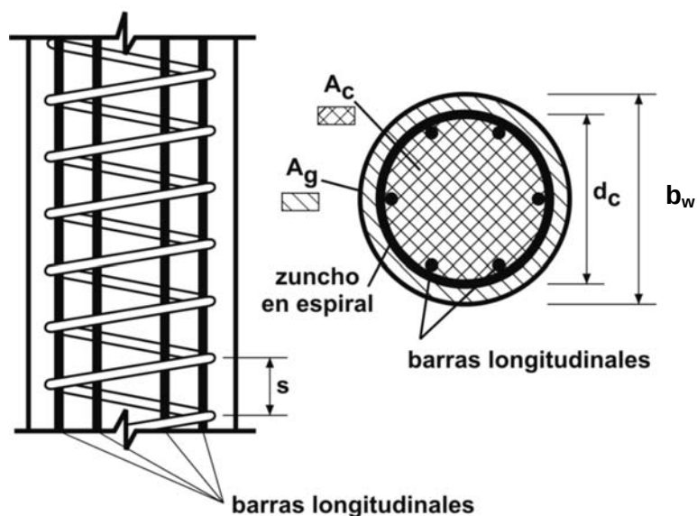
Figura 7.10.4.3. Armadura transversal en columnas (zunchos en espiral).
