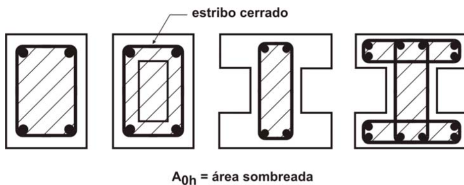
Figura 11.6.3.6. b) Definición de A_{0h} .
