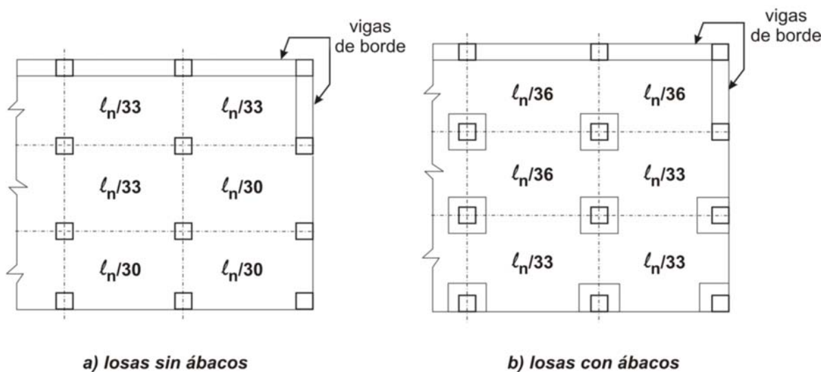
Figura 9.5.3.2. Ejemplo de espesor mínimo de las losas sin vigas interiores entre apoyos, con armadura f_y = 420 \text{ MPa} .
