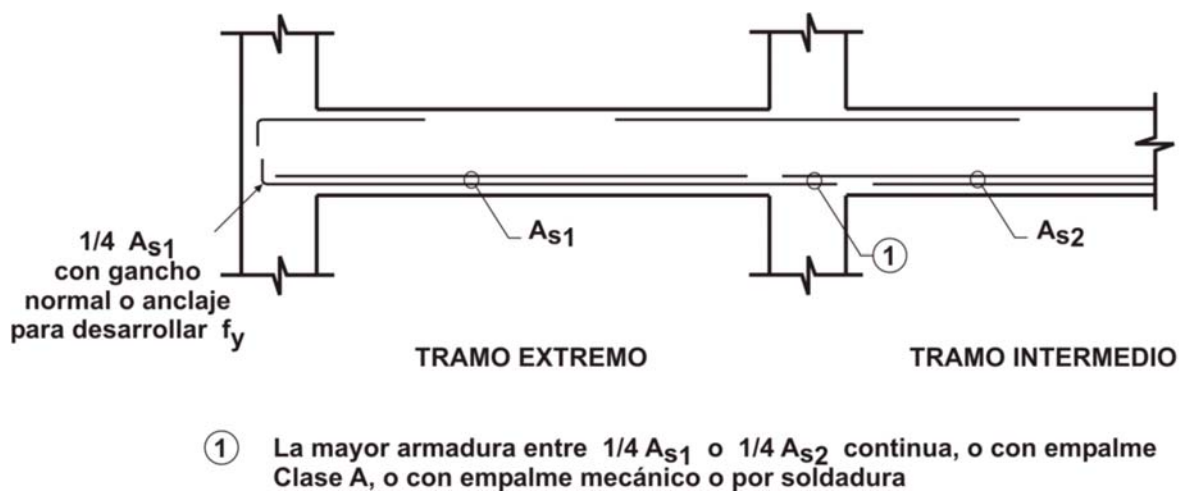
Figura 7.13.2.4. Armadura continua para vigas no perimetrales, sin estribos en U ni estribos cerrados (armadura requerida).
