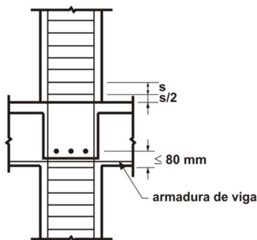
Figura 7.10.5.5. Terminación de los estribos cerrados para el caso de vigas en TODAS las caras de la columna.
