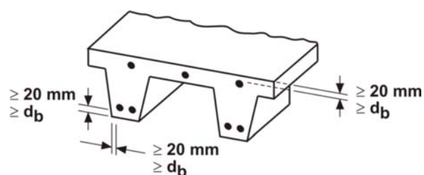
(c) Losas nervuradas no expuestas al aire libre ni en contacto con el suelo, con d_b \leq 32\text{ mm}
