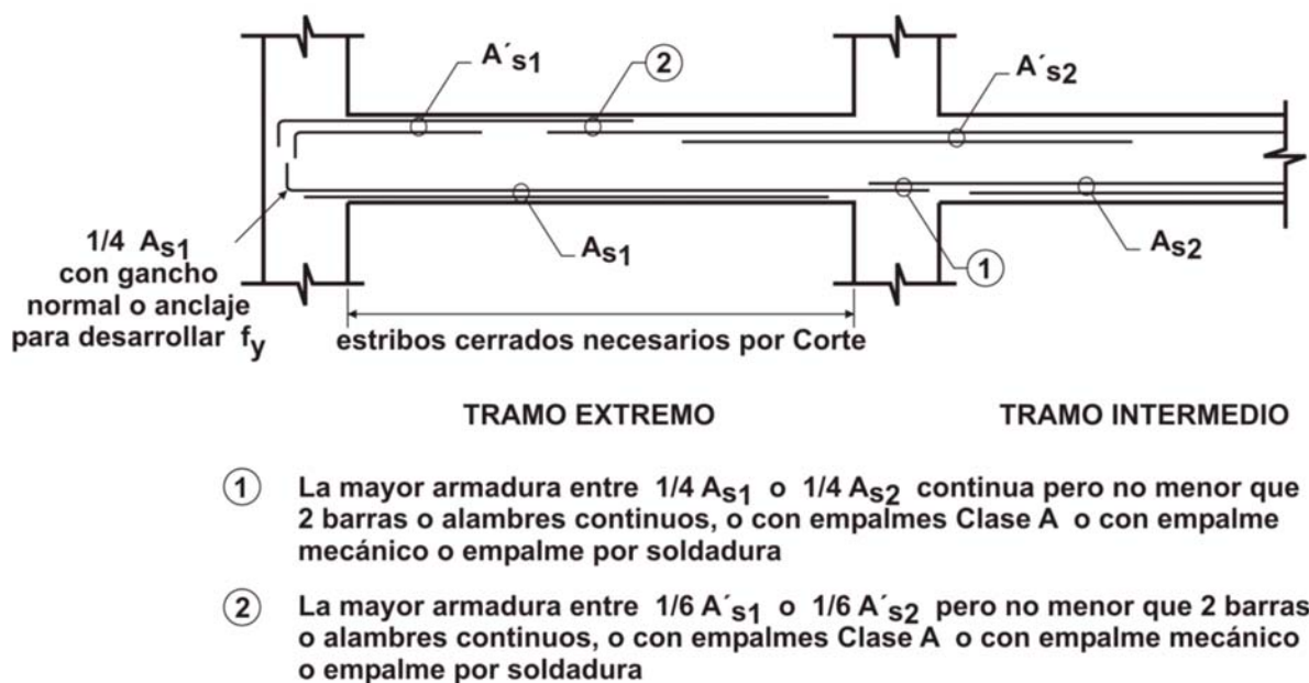
Figura 7.13.2.2. Armadura continua para vigas perimetrales (armadura requerida).
