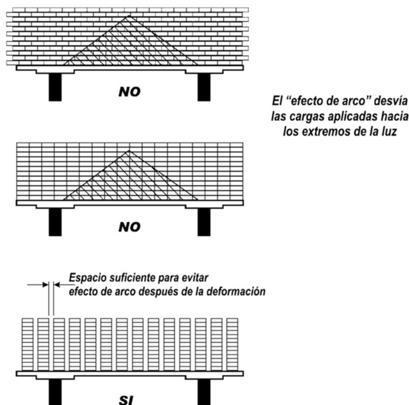
Figura 20.4.3. “Efecto de arco” y forma de evitarlo.
