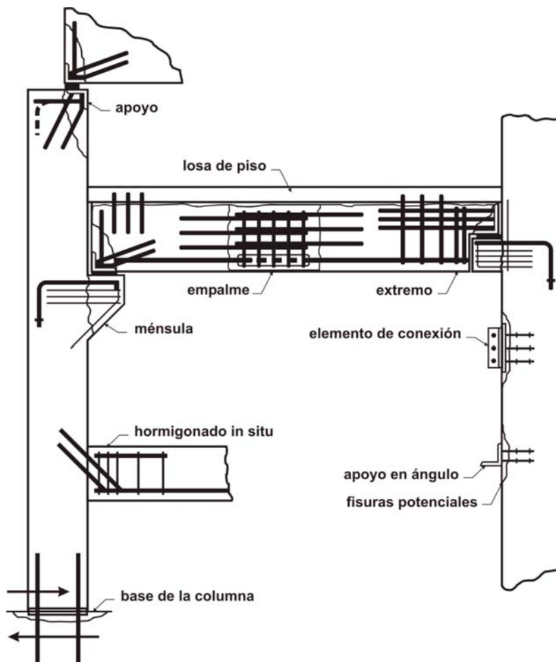
Figura 11.7.1. Aplicaciones del concepto de corte por fricción.
