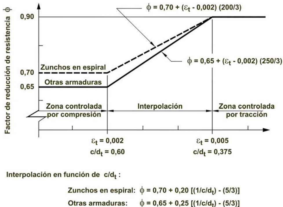
Figura 9.3.2. Ejemplo de variación de \phi en función de \epsilon_t y de la relación c/d_t para f_y = 420 MPa y para acero de pretensado. En los Comentarios a este artículo se presenta este gráfico para f_y = 500 MPa.
