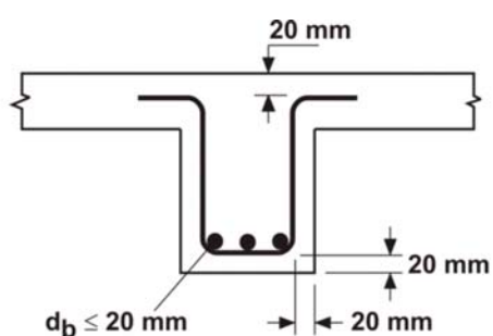
(c) Vigas no expuestas al aire libre ni en contacto con el suelo, con d_b \leq 20\text{ mm}
