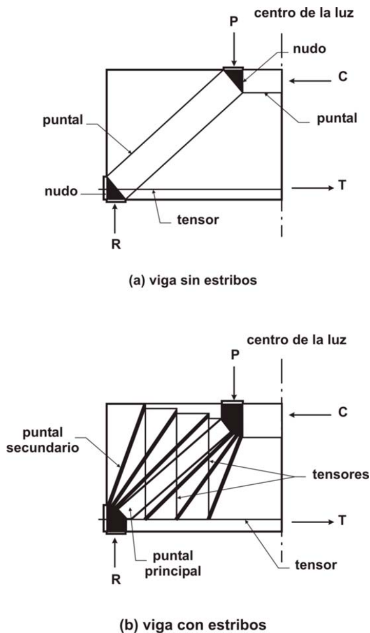
Figura 11.8.6.b). Modelos de armadura para vigas de gran altura. a) viga sin estribos; b) viga con estribos.
