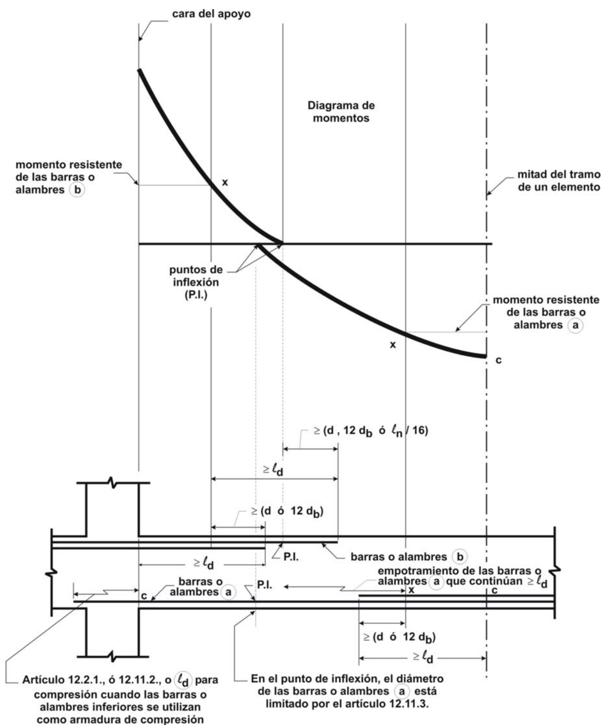
Figura 12.10.2. Anclaje de la armadura de flexión en una viga continua típica
