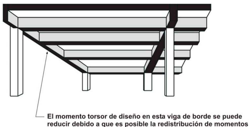
Figura 11.6.2.2. Ejemplo de momento torsor de diseño que se puede reducir. (ver el artículo 11.6.2.2.)
