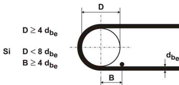
Figura 7.2.4.1. Doblado de una malla soldada con un mandril de diámetro < 8 d_b .
