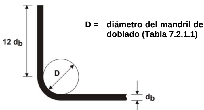
Figura 7.1.2. Gancho con un ángulo de doblado de 90° para barras y alambres de la armadura principal.
