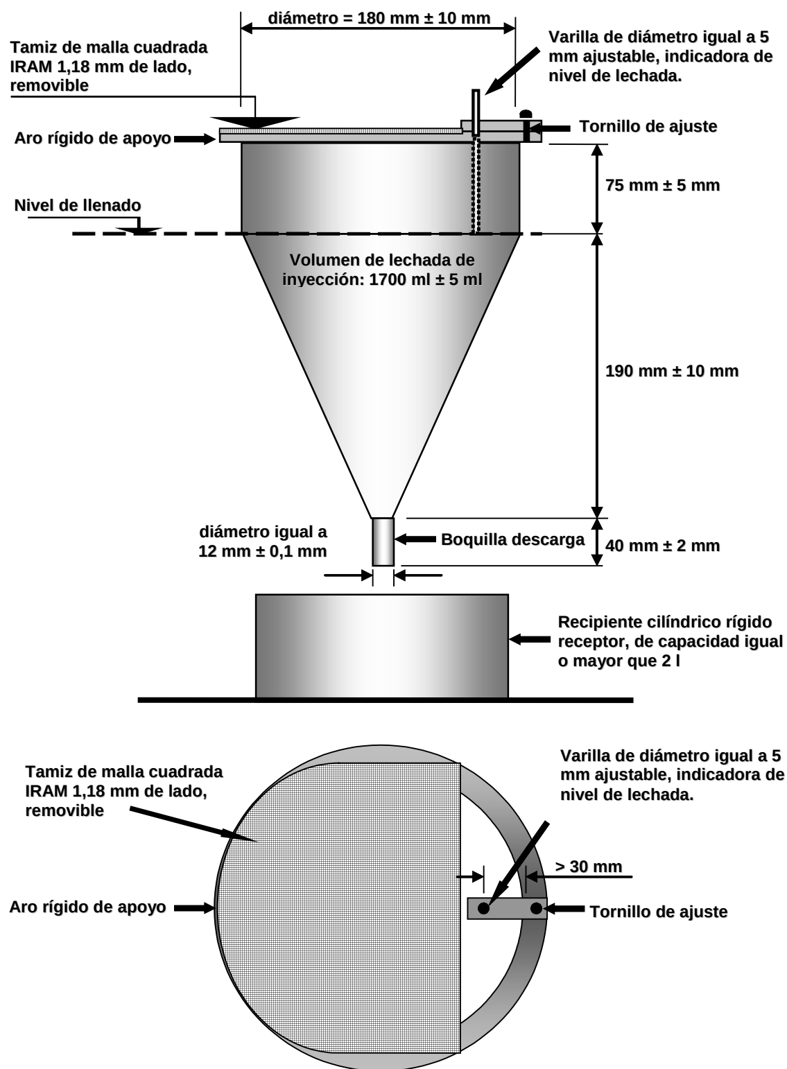
Figura 23.1. Cono de fluidez.
