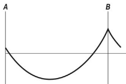
(d) momentos en las losas si la viga de borde es flexible a la torsión
