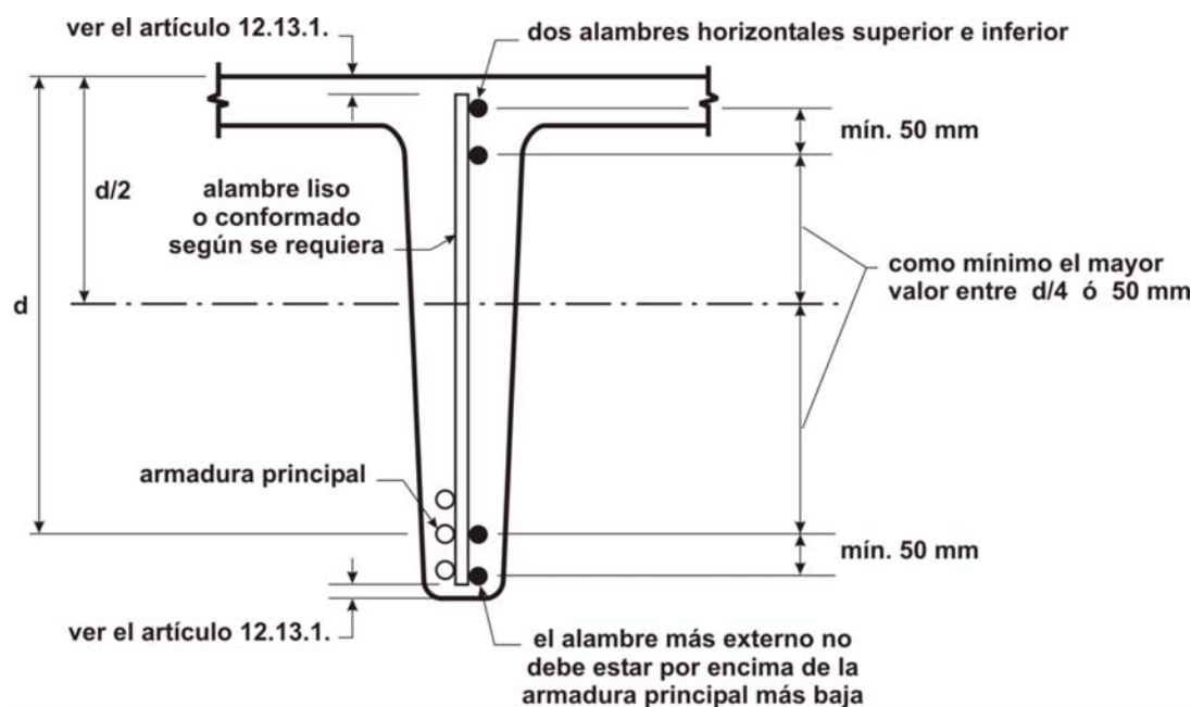
Figura 12.13.2.4. Anclaje de la armadura de corte compuesta por un estribo de una rama realizado con malla de acero soldada.
