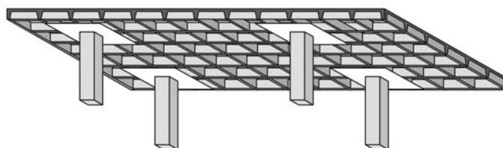
(d) Losa nervurada en dos direcciones
