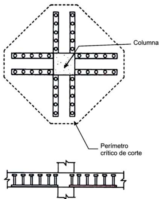
Figura 11.7.10. Armadura de corte constituida por pasadores con cabeza.
