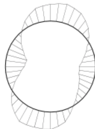
Momentos flexores
