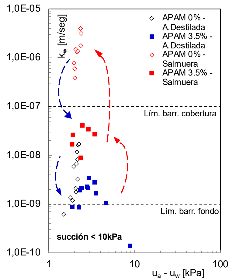
Variación de conductividad hidráulica no saturada por incorporación de APAM
