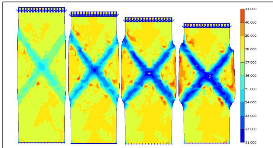
Localización deformaciones
