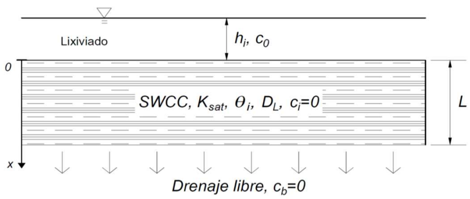
Modelo de infiltración 1D (advección + dispersión + difusión)
