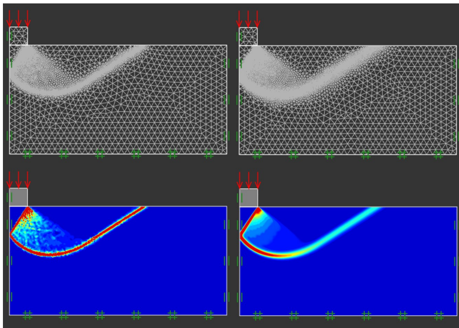
Determinación límites superior e inferior término N_\gamma para \phi=25^\circ (software OPTUM)
